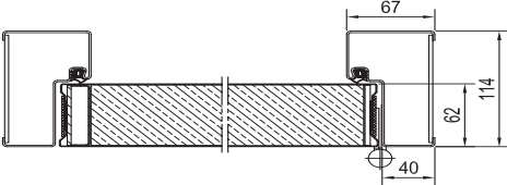
横剖视图
